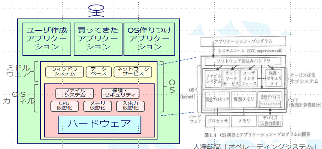
図1.1 オペレーティングシステムの構成
