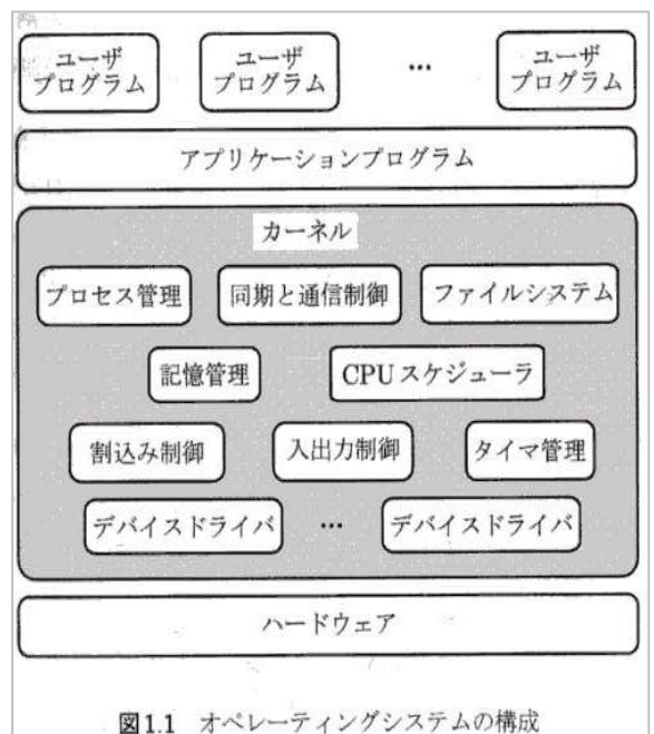
図1.1 オペレーティングシステムの構成
